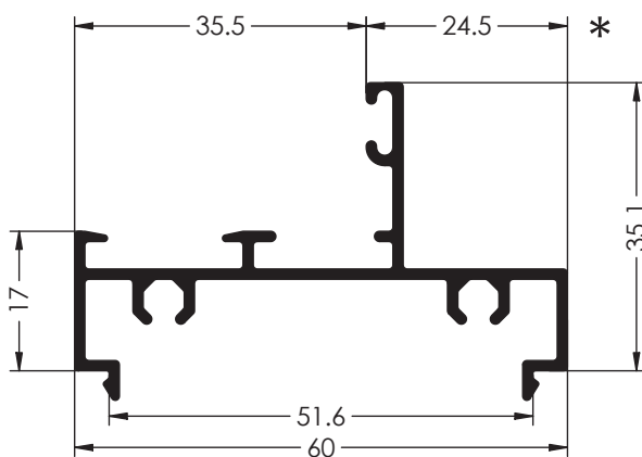
Ref. 6087 CERCO FIJO
