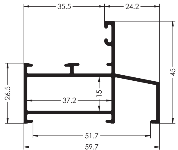
Ref. 6012 CERCO FIJO
