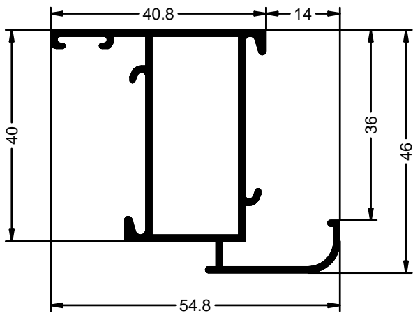
HOJA REDONDA
