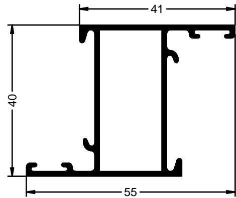
HOJA VENTANA
