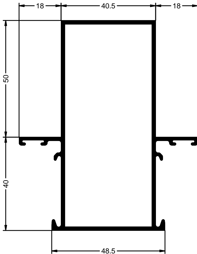
MURO CORTINA
