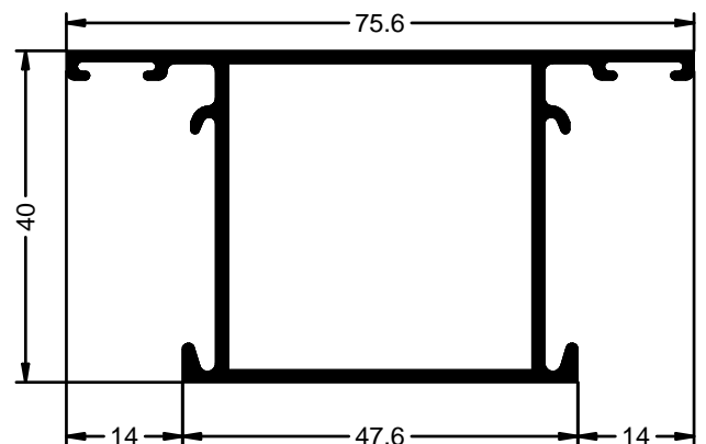
PILASTRA PUERTA
