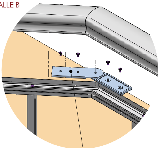
DETALLE B
