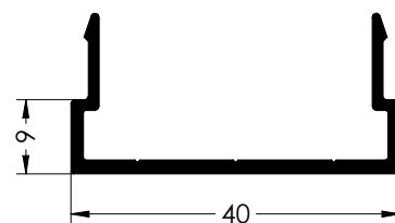
5211 - ANCLAJE "U"
