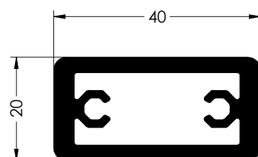
5212 - PIE 40x20
