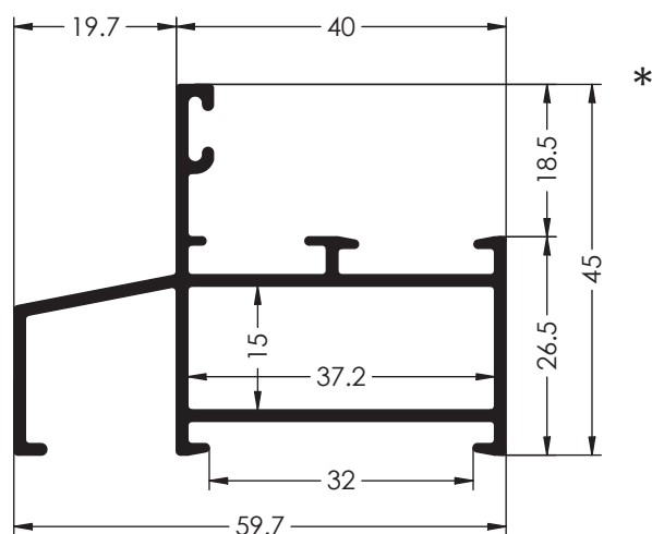
Ref. 6012 CERCO FIJO
