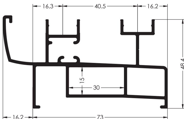
Ref. 6036 CERCO INFERIOR CONDENSACION
