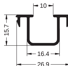
Ref. 6015 REDUCTOR CRISTAL SIMPLE
