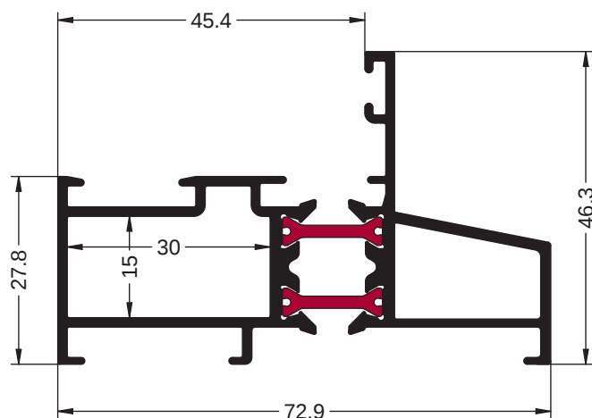
Ref. 9735 MARCOS FIJOS
