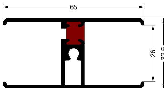
Ref. 9008 PARTE LUNAS
