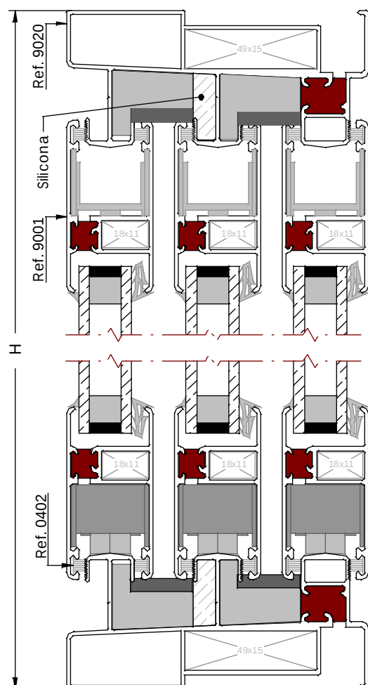
SECCIÓN VERTICAL
