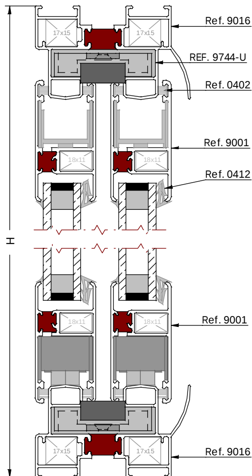
SECCIÓN VERTICAL
