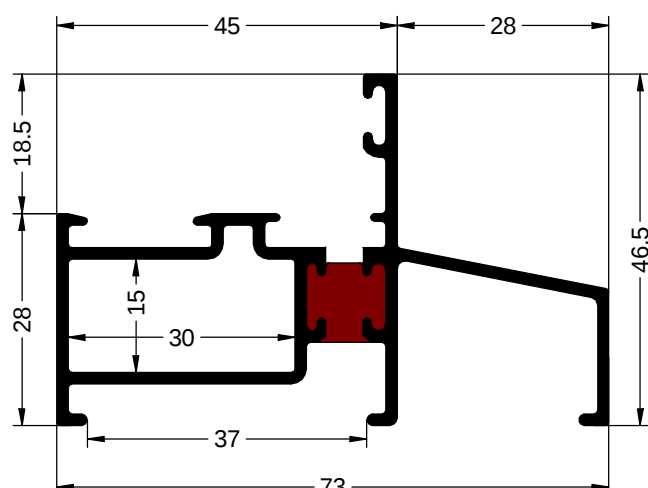
Ref. 9003 CERCO FIJO
