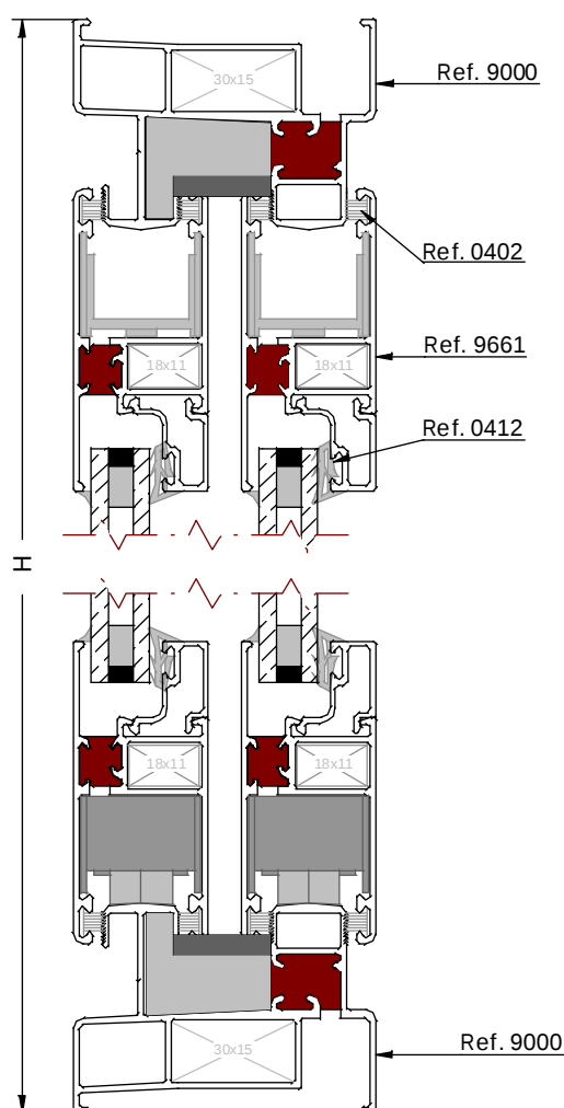
SECCIÓN VERTICAL 1:2
