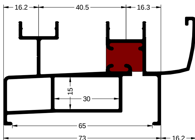
Ref. 9036 CERCO INFERIOR CONDENSACION
