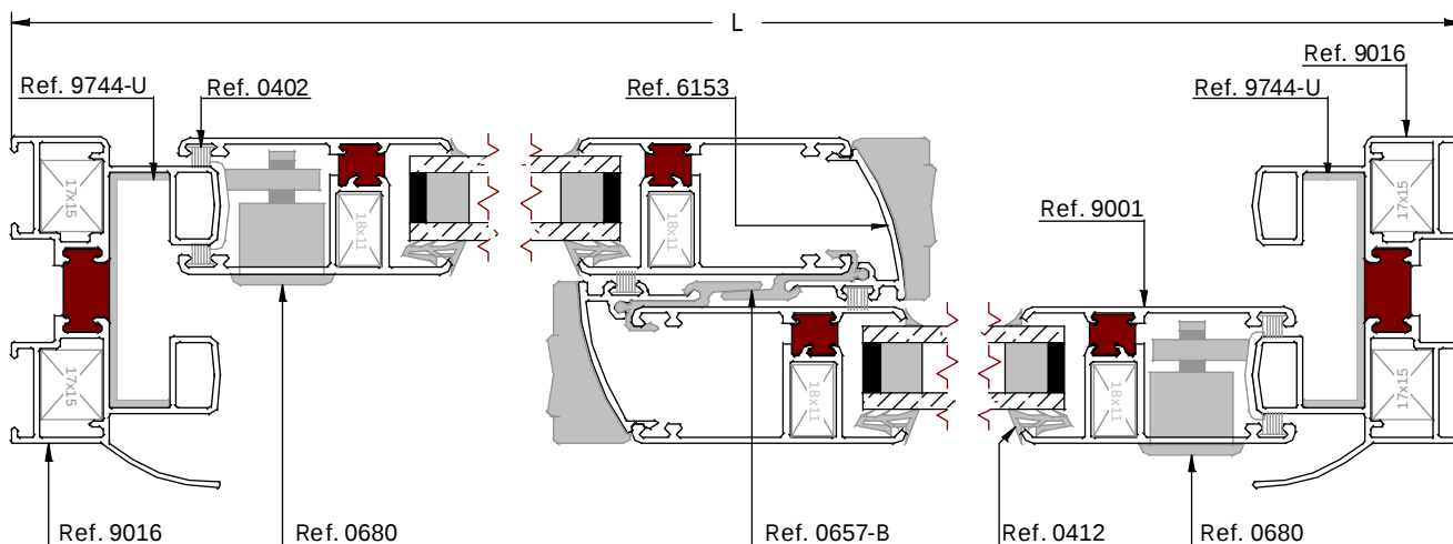
SECCIÓN HORIZONTAL
