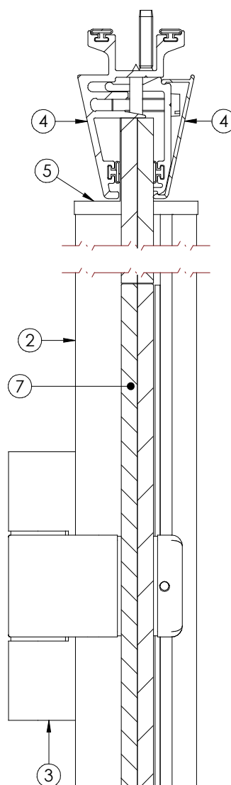
CORTE J-J 1:2
