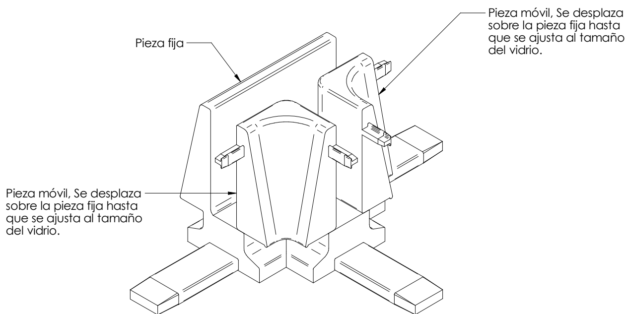
Detalle del Nudo "T". REF.0049-T
