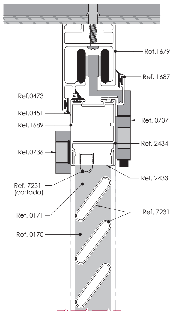
Sección Vertical Lama Fija
