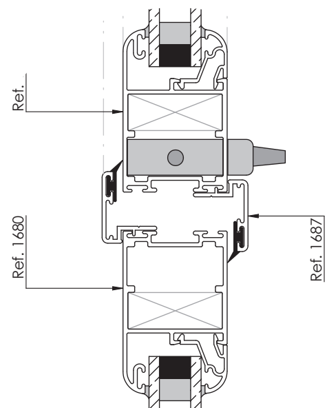
DETALLE B 1:2
