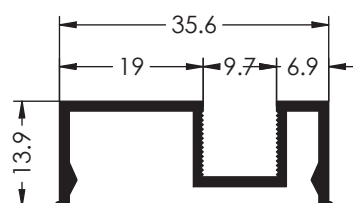
Ref. 2433 REMATE INFERIOR Y SUPERIOR MALLORQUINAS
