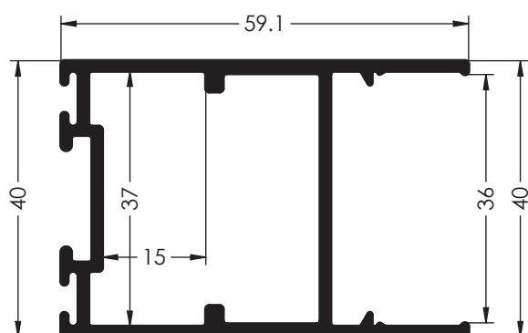
Ref. 1689 HOJA MALLORQUINAS
