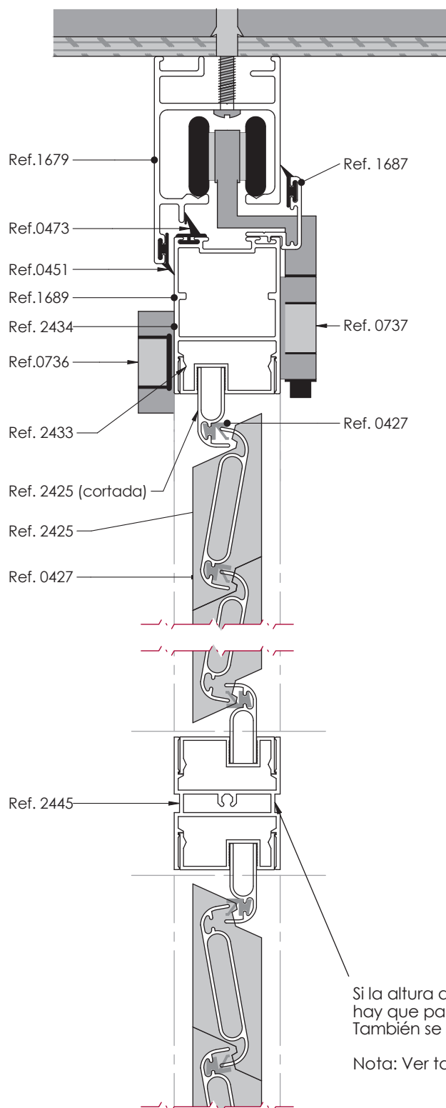
Sección Vertical Lama Orientable
